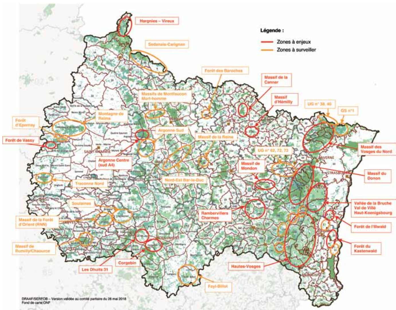
Carte du zonage des secteurs identifiés au titre de l'équilibre sylvo-cynégétique (Source : DRAAAF/SERFOB)
